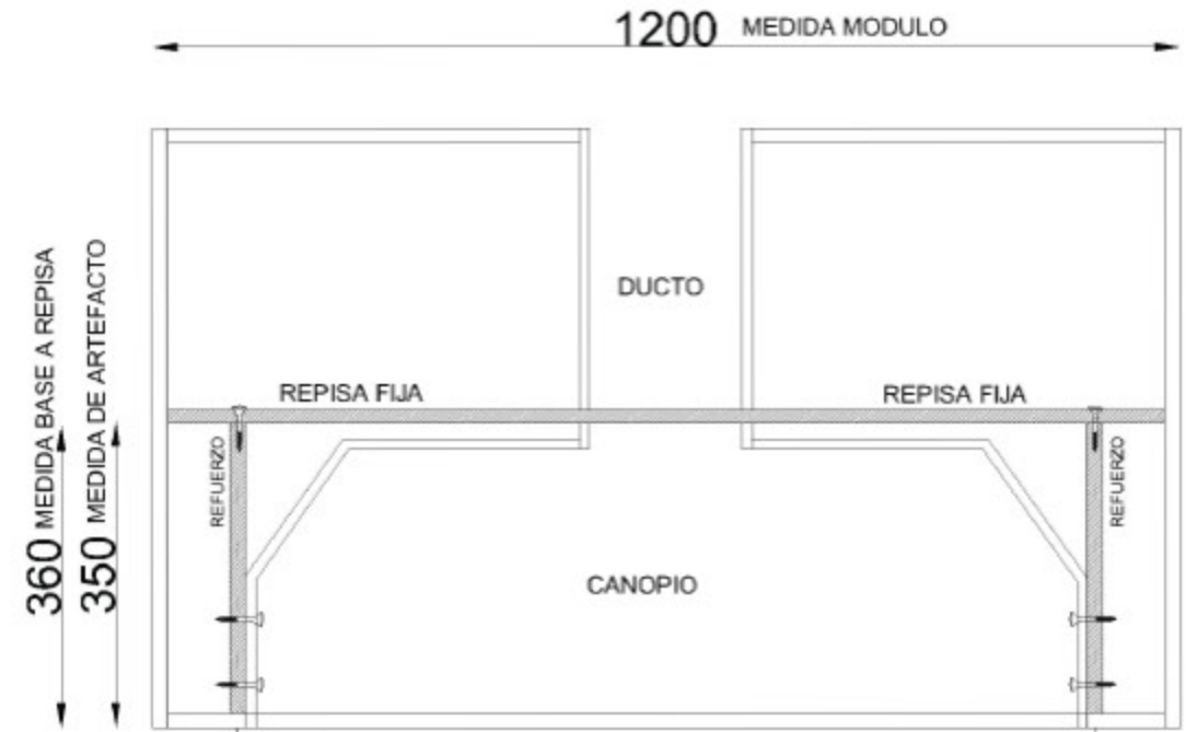
CORTE DELANTERO, PARA MÓDULO > 1020MM (MEDIDAS EN MM)
