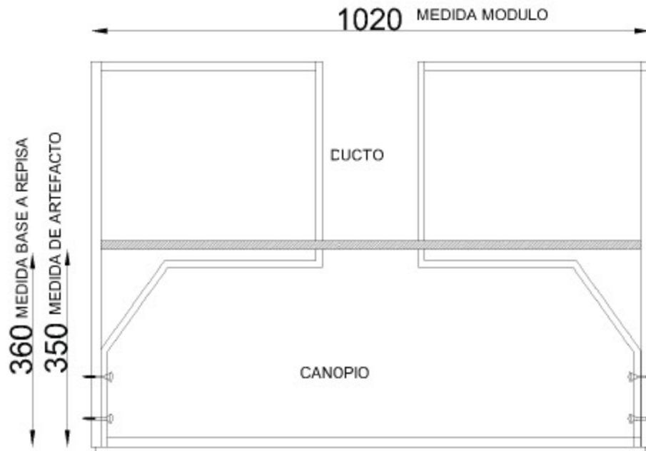
CORTE DELANTERO, PARA MÓDULO 1020MM (MEDIDAS EN MM)
